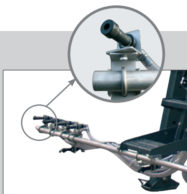
Hochgeschwindigkeitsstreuern mit Spratronic-Düsen.
