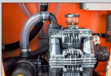
Logisch aufgebautes Solesystem mit Membranpumpe.
